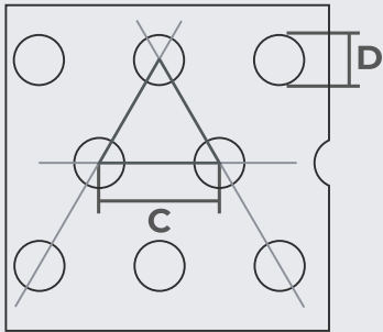
TRABADO A 60°
