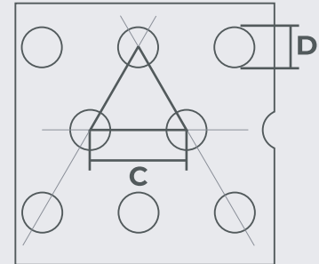
TRABADO A 60°
